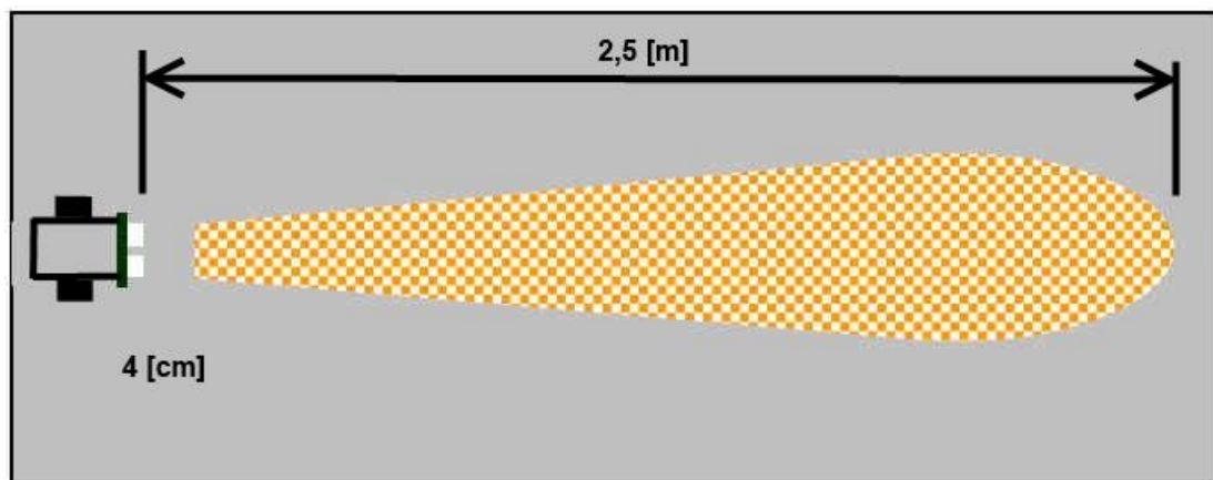
Slika 3.23 Prikaz udaljenosti u obliku konusa za ultrazvučni senzor
