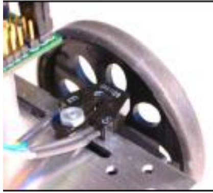
Slika 3.25 Prikaz korištenja infracrvenog fotoreflektivnog senzora za praćenje kretnje kotača mobilnog robota
