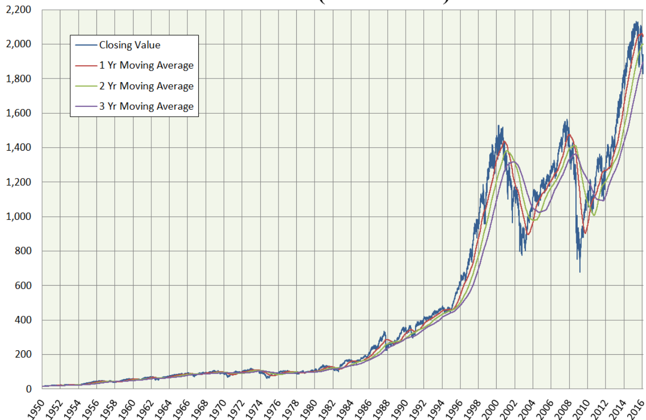
Slika 4. S&P 500 indeks (1950 - 2016)
