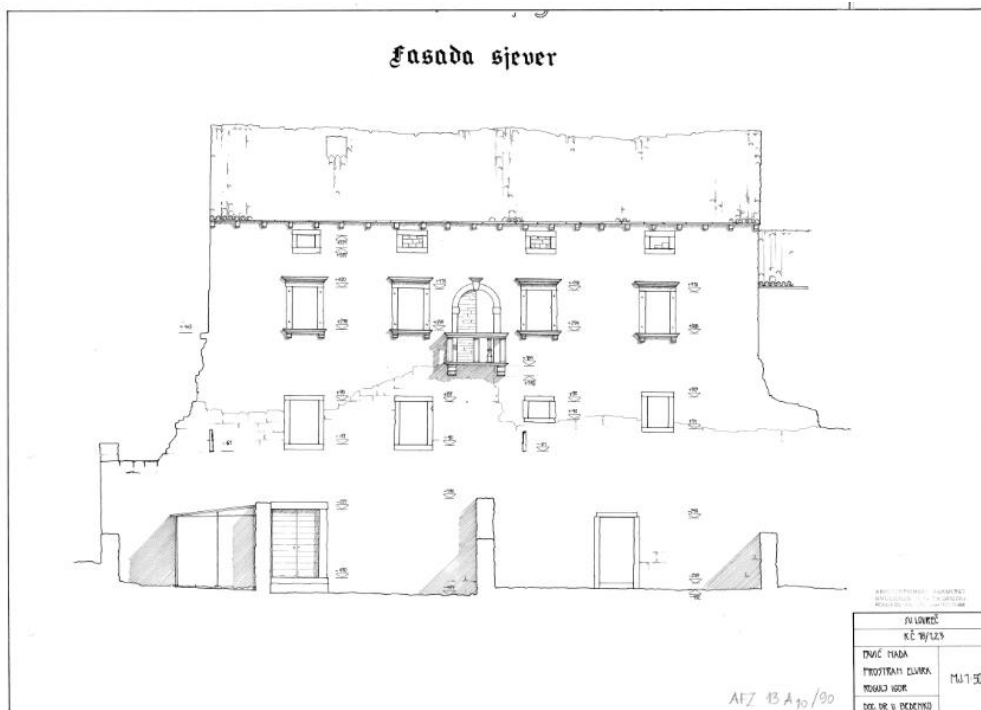
Slika 25. Arhitektonska snimka sjevernog pročelja kuće Frigerio, autora: N. Pavić, E. Prostran, I. Rogulj (projekt dr. sc. V. Bedenka)
