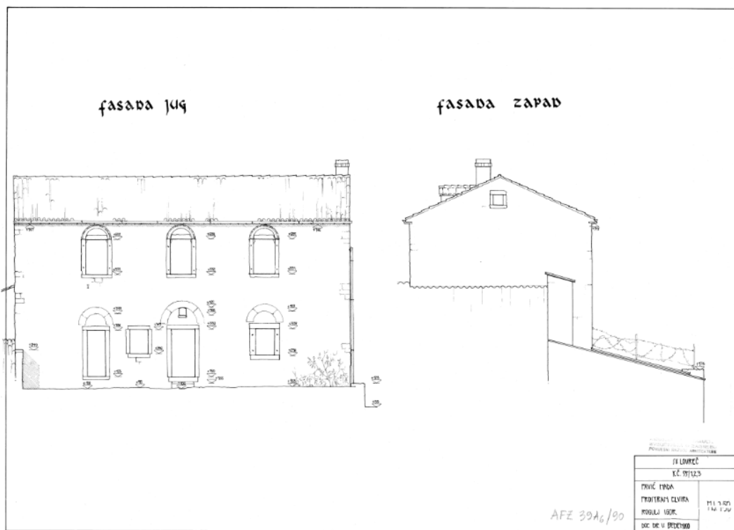
Slika 21. Arhitektonska snimka južnog i zapadnog pročelja Kapetanove kuće, autora: N. Pavić, E. Prostran, I. Rogulj (projekt dr. sc. V. Bedenka)
