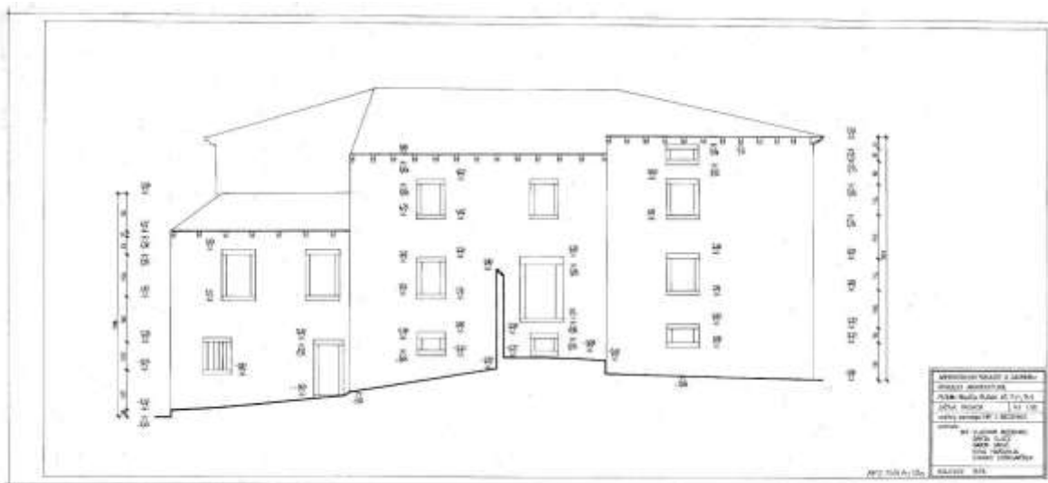
Slika 112. Plomin, palača Rudan, 18. st, južna fasada, kotirani arhitektonski snimak. Izradili: V. Bedenko, G. Glatz, D. Grgić, N. Haramija, S. Stergaršek (Arhitektonski fakultet u Zagrebu, 1978.)
