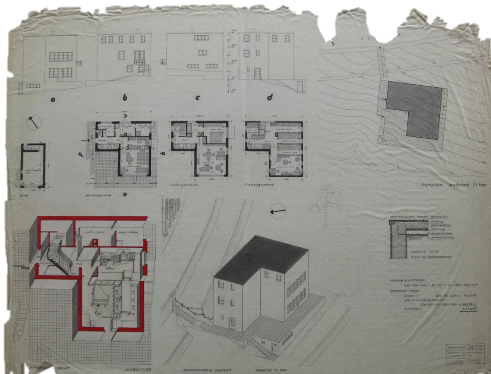
136. Reinhold Rossig, entwurf: einfamilienhaus in pilsnitz bei drd., 01.06.1932, Stiftung Bauhaus Dessau: I 5721 G
