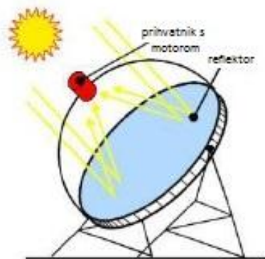
Sl.3.14. Koncept koncentriranja sunčevih zraka kod tanjurastog paraboličnog kolektora [22]
