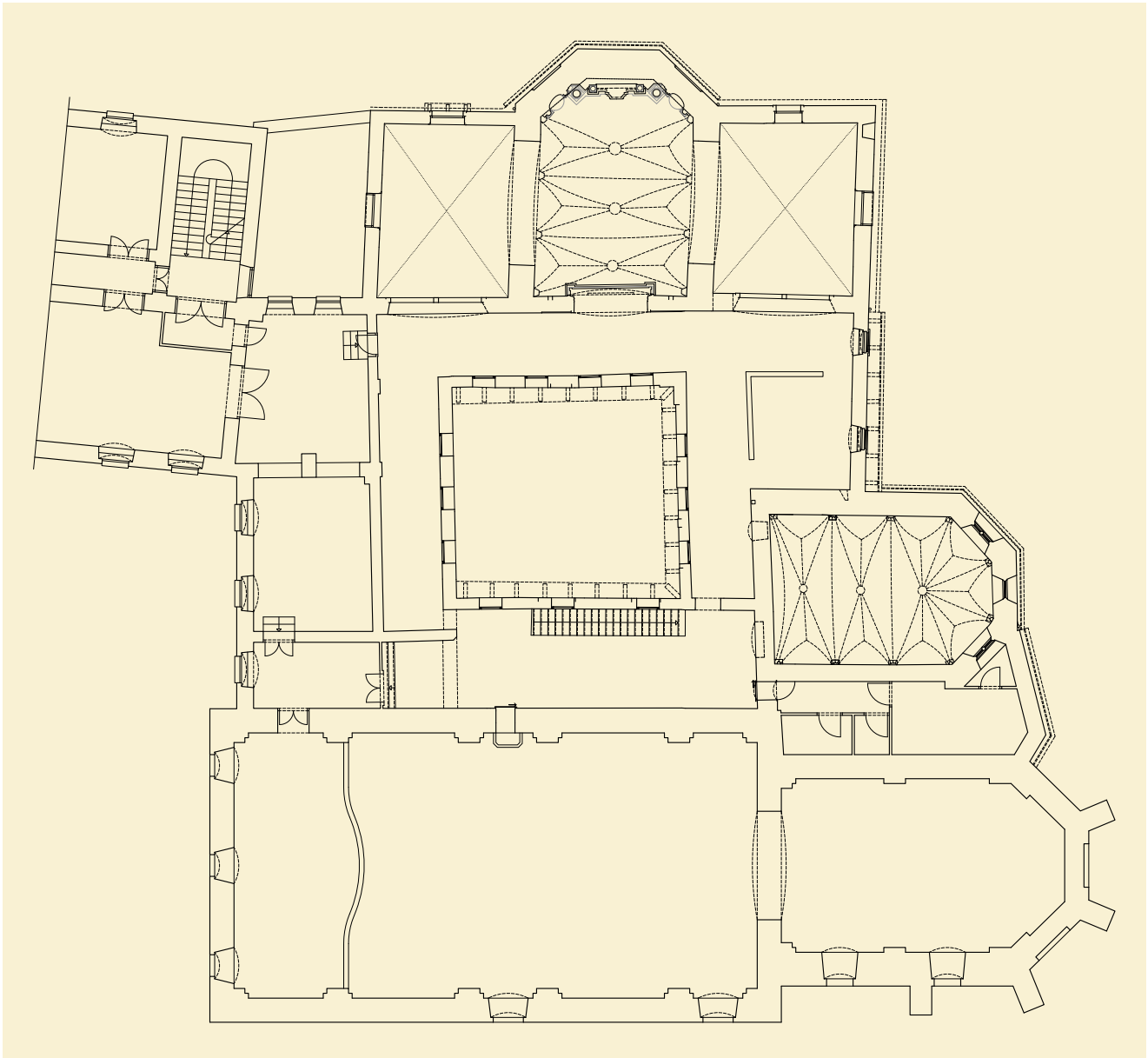
4. Rijeka, tlocrt jezgre nekadašnjega augustinskog samostana u razini kata (nije prikazano historicističko stubište pridodano klausturu i dio recentnoga zida samostana), (izradili: mr. sc. A. Braun d. i. a., M. Cvitanović d. i. a., V. Lukić d. i. a., T. Vidović d. i. a., Zavod za arhitektonsko nasljeđe Arhitektonskog fakulteta Sveučilišta u Zagrebu)
