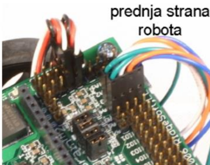
Slika 3.11 Spajanje senzora za kretanje kotača na upravljački kontroler
