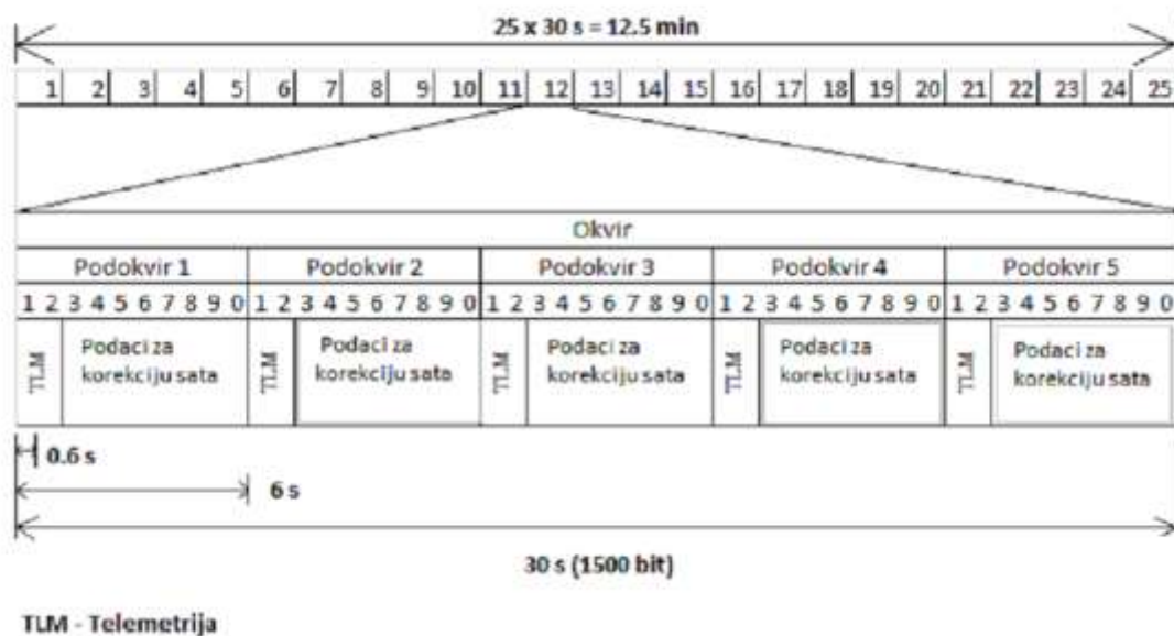
Slika 2.4. GPS signal
