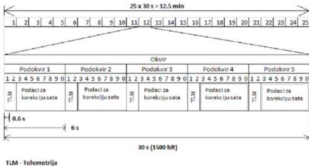
Slika 2.4. GPS signal
