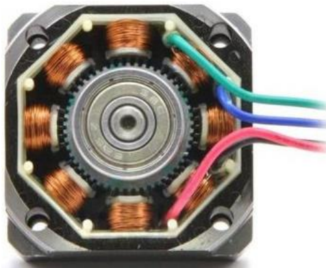
Slika 3.12. Koračni motor.
