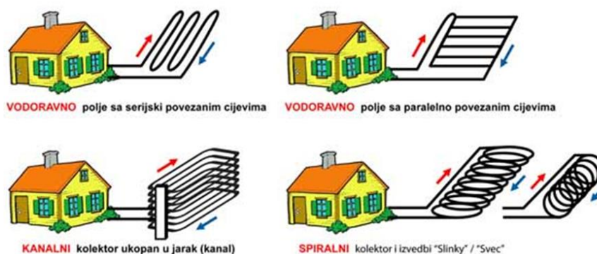
Slika 8: Izvedbe zatvorenog sustava s podzemnim kolektorima [9]
