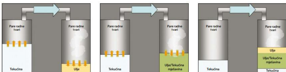
Slika 13: Kondenziranje radne tvari unutar kompresora [25]
