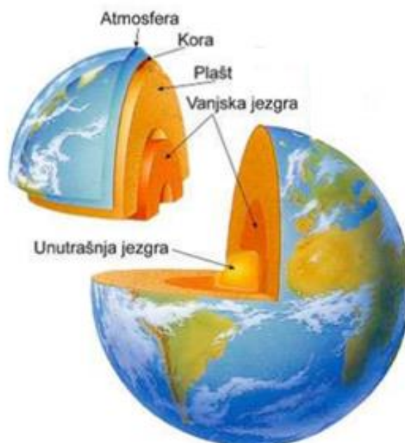
Slika 1: Presjek Zemlje [1]
