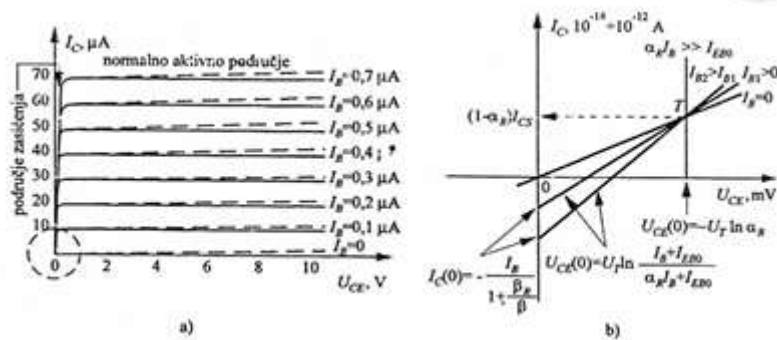
Slika 3.2 Izlazne karakteristike u spoju zajedničkog emitera tranzistora : a) za idealni tranzistor (puna crta), za realni tranzistor (isprekidana crta ) b) uvećano područje oko ishodišta
