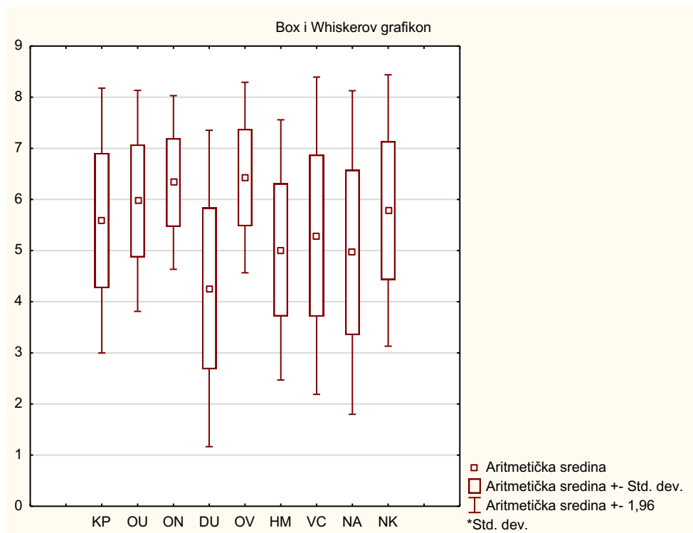
Slika 47 – Box i Whiskerov grafikon aritmetičke sredine, aritmetičke sredine \pm standardne devijacije i aritmetičke sredine \pm 1,96 *standardna devijacija uzorka ankete za internetske portale i aplikacije
