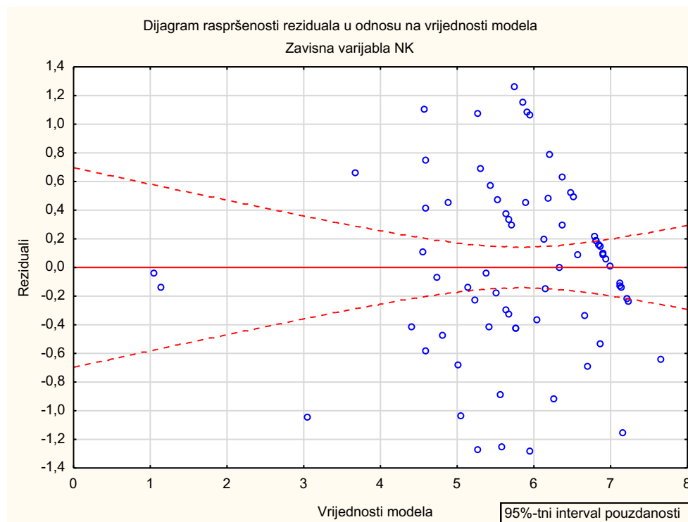
Slika 55 – Dijagram raspršenosti reziduala i vrijednosti konačnog linearnog regresijskog modela varijable INT_NK i nezavisnih varijabli za internetske portale i aplikacije
