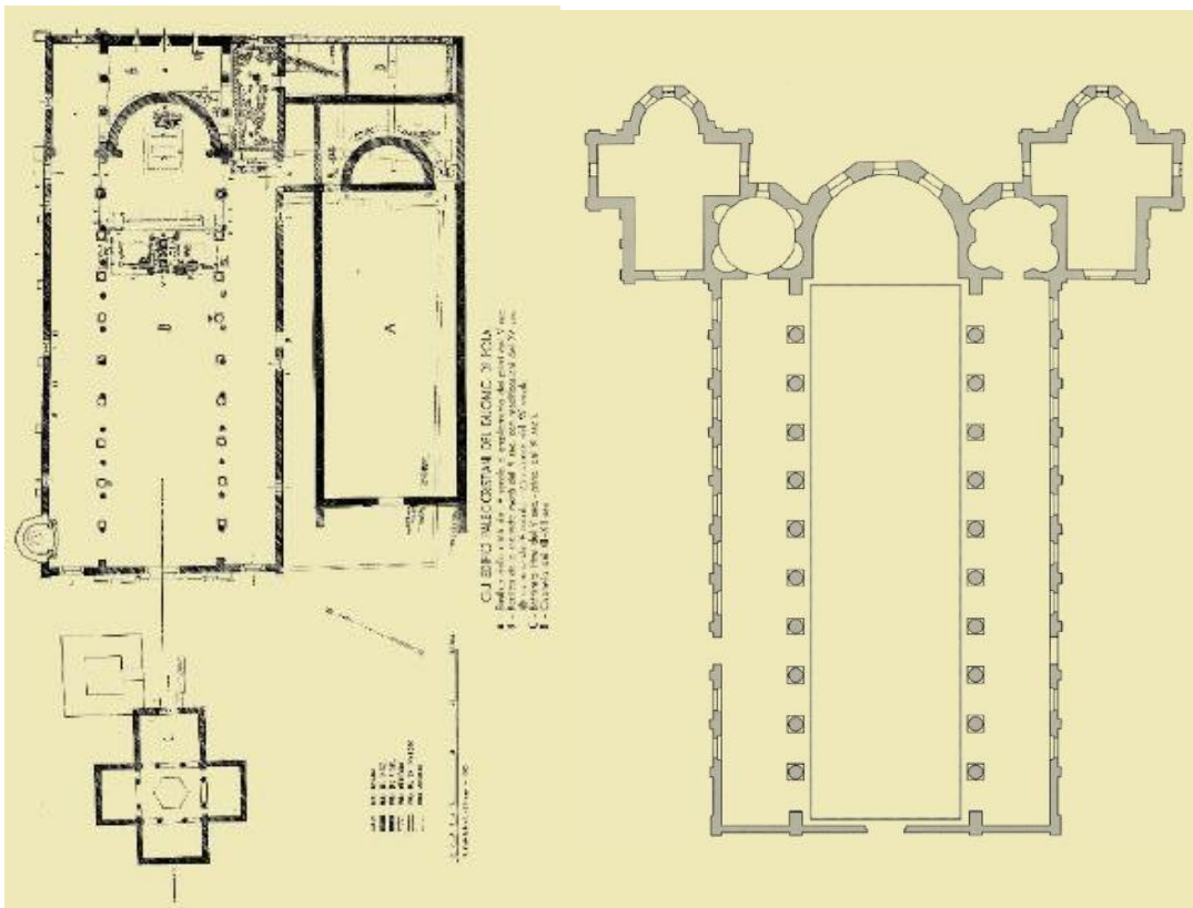
Slika 3. Katedrala u Puli, sveta Marija Formoza u Puli
