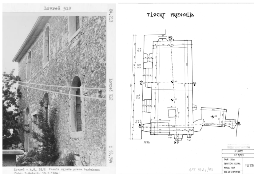
Slika 17. i 18. „Fasada zgrade prema barbakamu“ (južno pročelje Kapetanove kuće) D. Grigić, 1994. (Fototeka Konzervatorskog odjela u Rijeci) i tlocrt prizemlja Kapetanove kuće, autora: N. Pavić, E. Prostran, I. Rogulj (projekt dr. sc. V. Bedenka)
