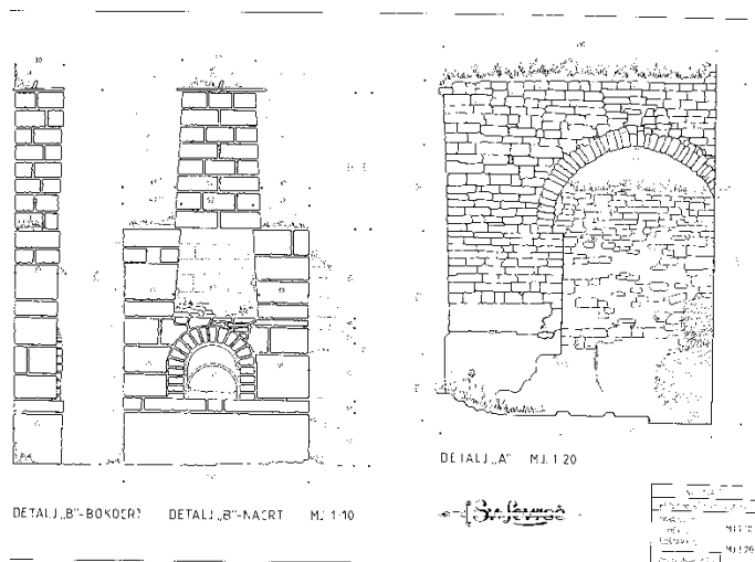
Slika 4. i 5. Romanička vrata, snimila: Irena Radoslav, 2021. i arhitektonska snimka Romaničkih vrata, autora: D. Dobrinić, G. Juričić, S. Šoštarić, 1982.-1983. (projekt doc. dr. V. Bedenka)
