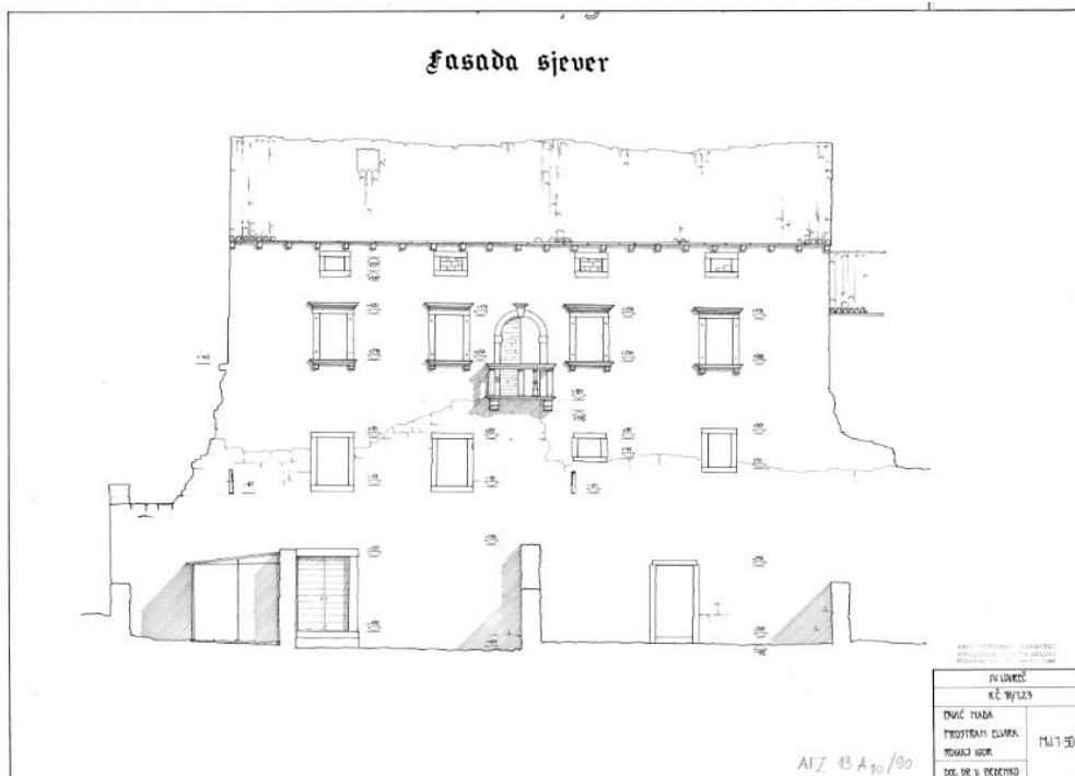
Slika 25. Arhitektonska snimka sjevernog pročelja kuće Frigerio, autora: N. Pavić, E. Prostran, I. Rogulj (projekt dr. sc. V. Bedenka)
