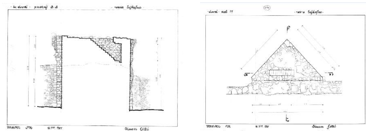
Slika 7. Arhitektonska snimka Trokutaste kule, autora: T. Gottel, 1988. (projekt doc. dr. V. Bedenka)
