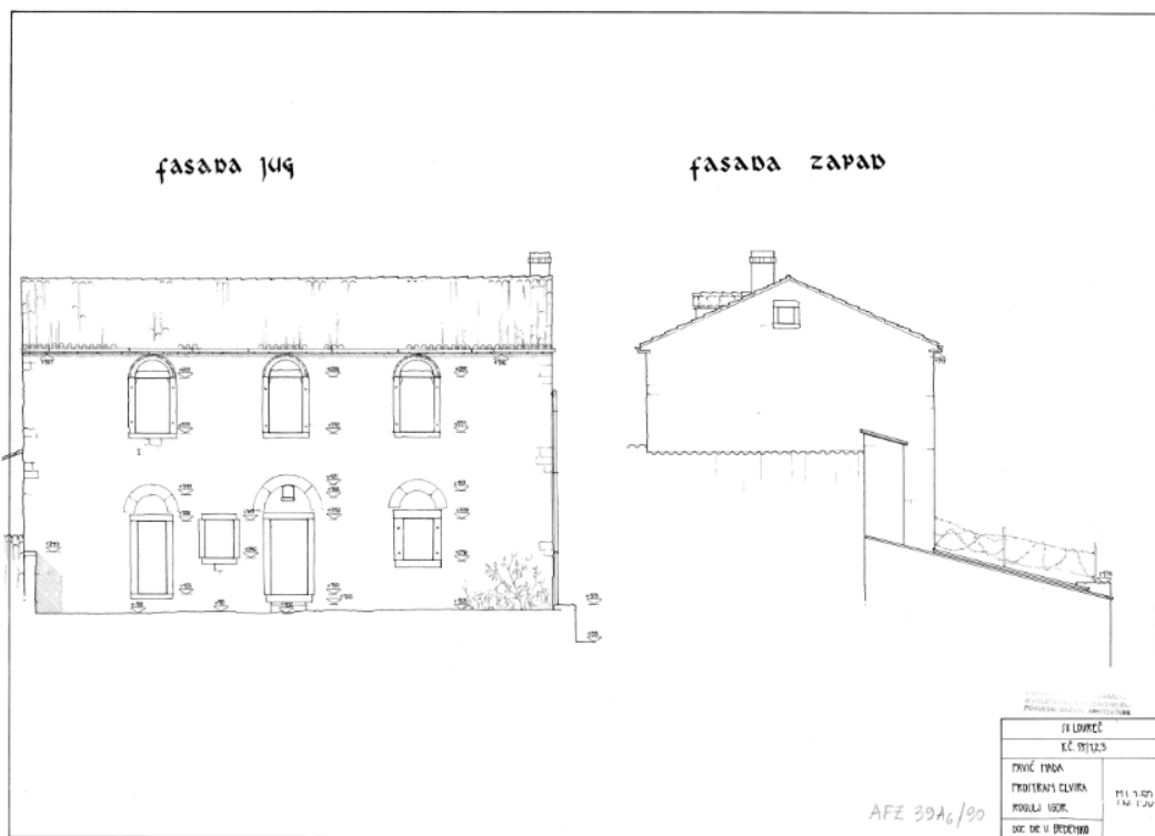
Slika 21. Arhitektonska snimka južnog i zapadnog pročelja Kapetanove kuće, autora: N. Pavić, E. Prostran, I. Rogulj (projekt dr. sc. V. Bedenka)
