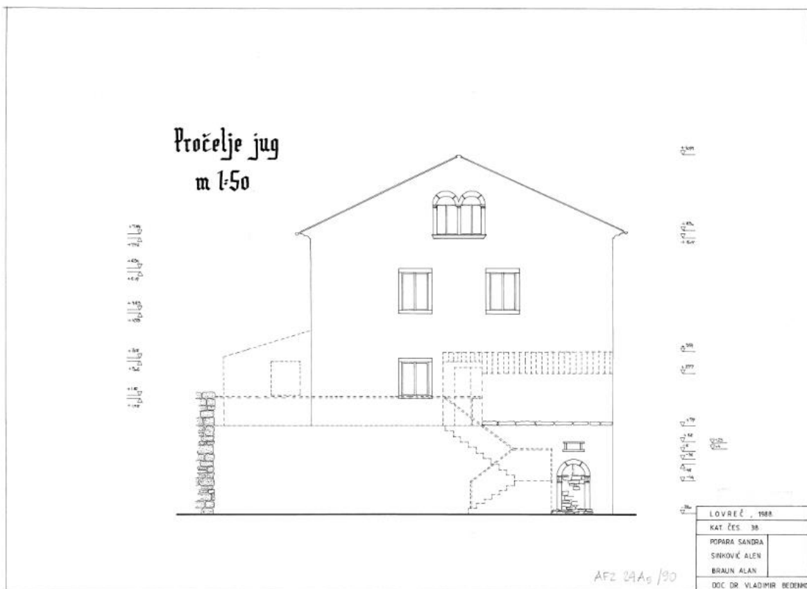
Slika 33. Arhitektonska snimka južnog pročelja kuće na k.č. 38, autora: S. Popara, A. Sinković, A. Braun (projekt dr. sc. Vladimira Bedenka), 1988.
