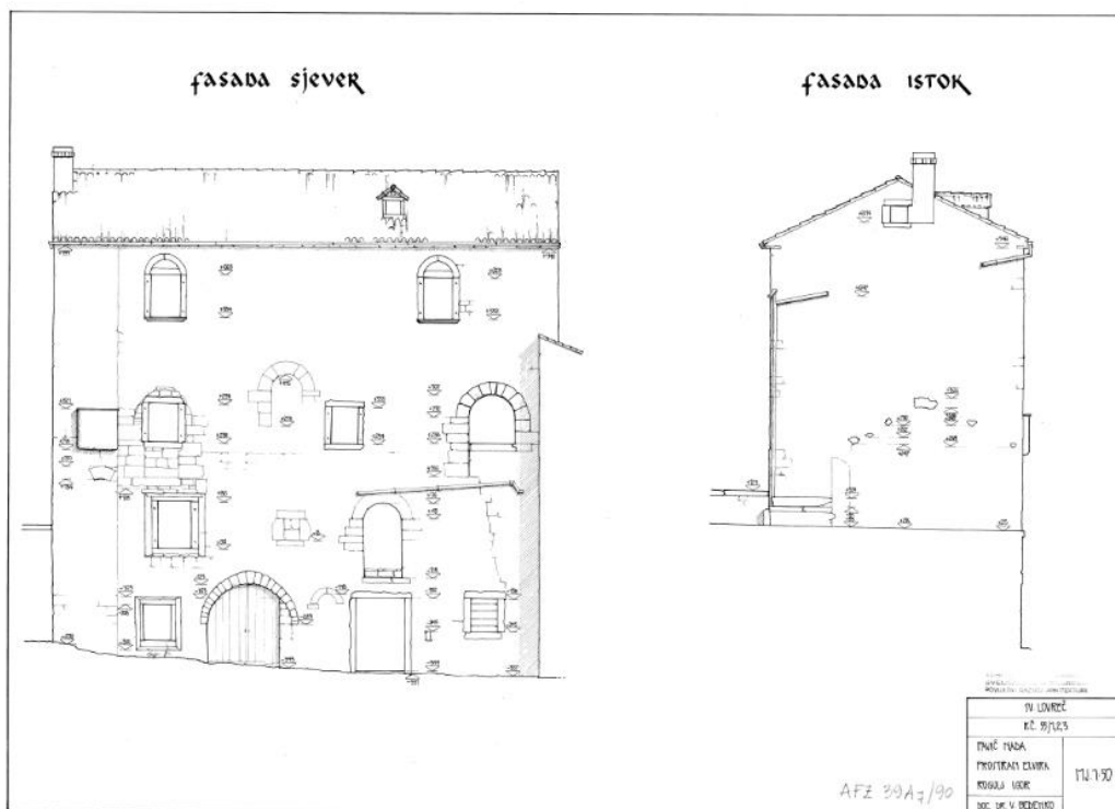
Slika 20. Arhitektonska snimka sjevernog i istočnog pročelja Kapetanove kuće, autora: N. Pavić, E. Prostran, I. Rogulj (projekt dr. sc. V. Bedenka)
