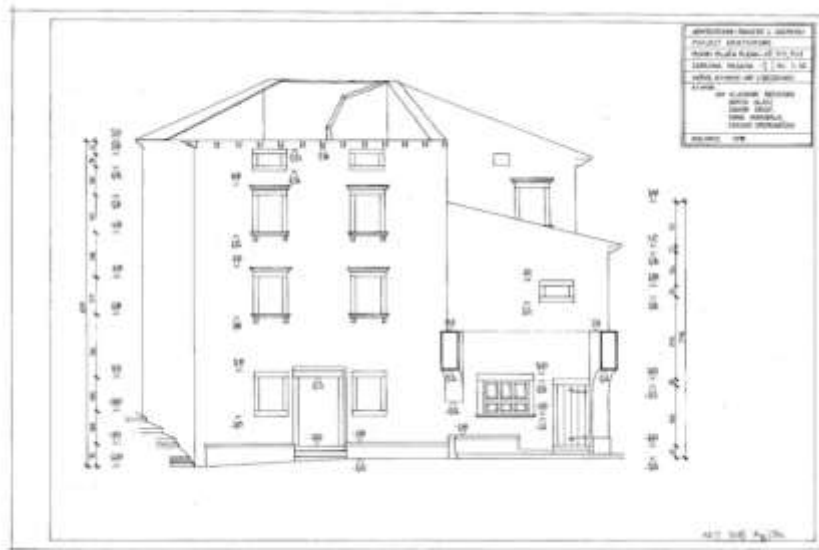
Slika 113. Plomin, palača Rudan, 18. st, zapadna fasada, kotirani arhitektonski snimak. Izradili: V. Bedenko, G. Glatz, D. Grgić, N. Haramija, S. Stergaršek (Arhitektonski fakultet u Zagrebu, 1978.)
