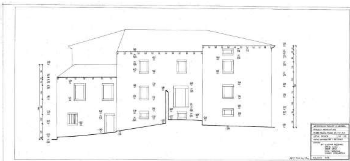
Slika 112. Plomin, palača Rudan, 18. st, južna fasada, kotirani arhitektonski snimak. Izradili: V. Bedenko, G. Glatz, D. Grgić, N. Haramija, S. Stergaršek (Arhitektonski fakultet u Zagrebu, 1978.)
