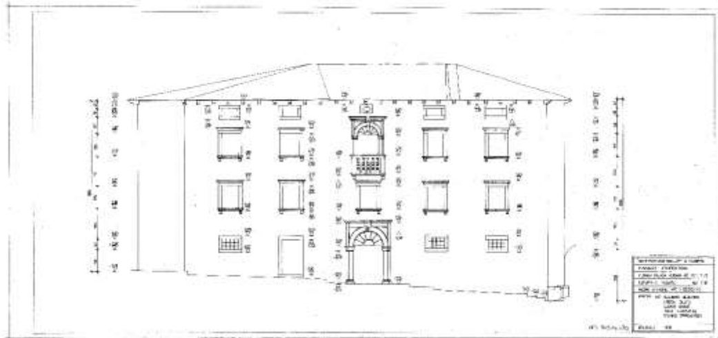
Slika 106. Plomin, palača Rudan, 18. st, sjeverna fasada, kotirani arhitektonski snimak. Izradili: V. Bedenko, G. Glatz, D. Grgić, N. Haramija, S. Stergaršek (Arhitektonski fakultet u Zagrebu, 1978.)
