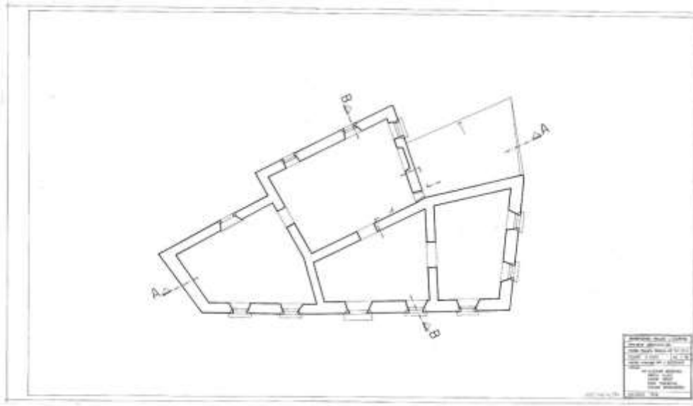
Slika 111. Plomin, 18. st, palača Rudan, tlocrt drugog kata. Izradili: V. Bedenko, G. Glatz, D. Grgić, N. Haramija, S. Stergaršek (Arhitektonski fakultet u Zagrebu, 1978.)
