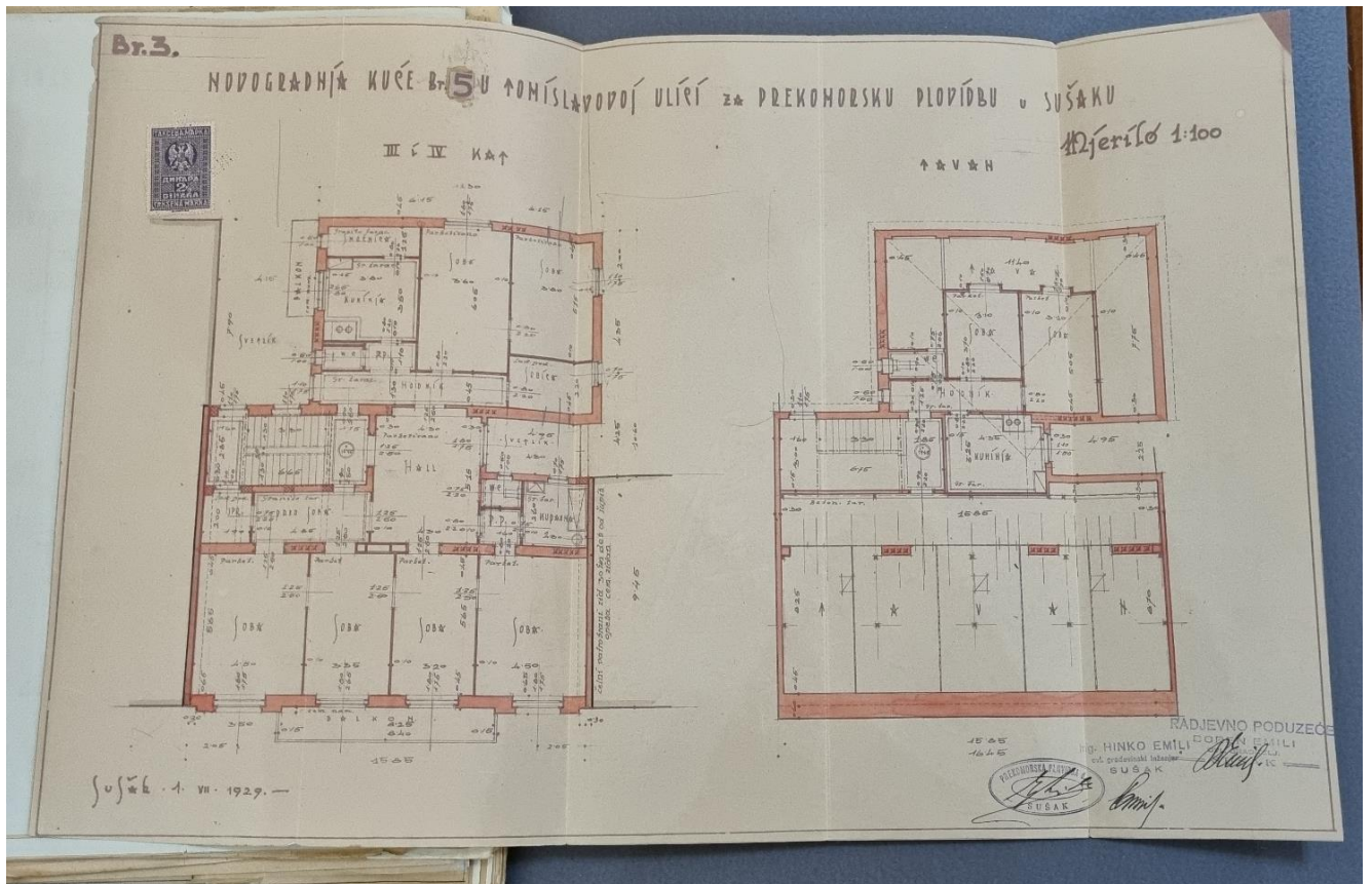
(Slika 7. Tlocrt trećeg i četvrtog kata te tavana zgrade Prekomorske plovidbe, 1929., HR-DARI-58, kut. 11/108, foto Gracia Valent)
