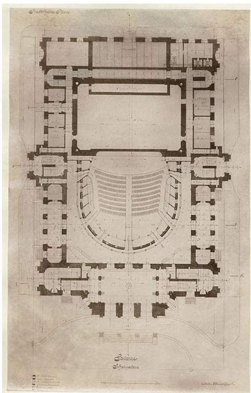
Prilog 3.2.4, Tlocrt kazališne zgrade, izvor: http://www.muzej-rijeka.hr/akvizicije-2006-2010/zbirka-filmske-i-kazalisne-gradje.html
