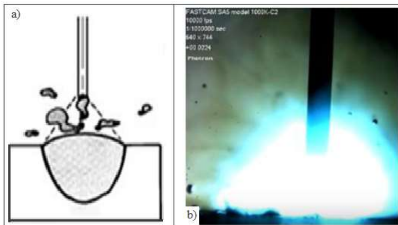
Slika 2.30. Prikaz krupnokapljicastog režima rada, a) shema, b) fotografija [9, 15]
