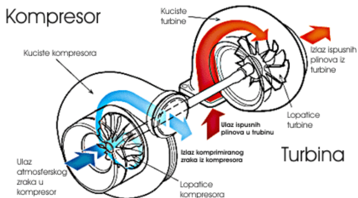
Slika 4.45. Dijelovi turbopuhala
