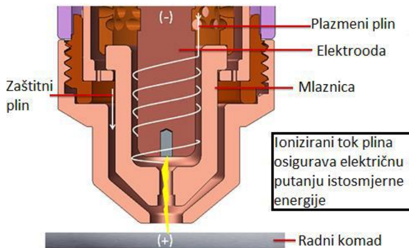
Slika 2.7. Putanja plazmenog luka do radnog komada [6]
