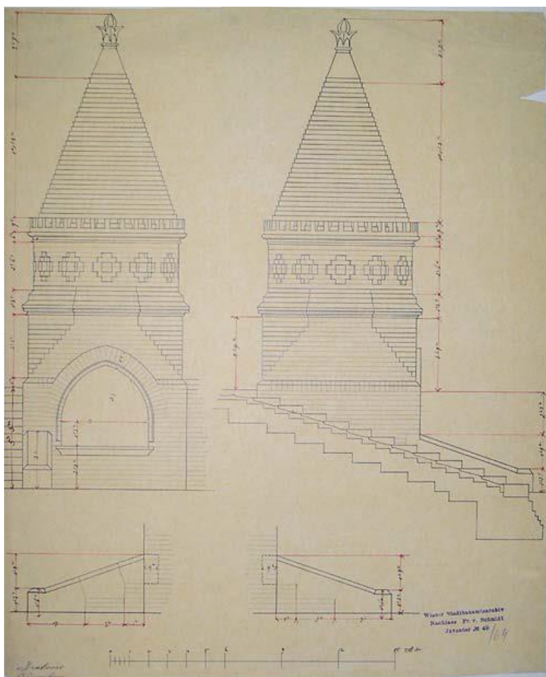
Slika 9. Friedrich Schmidt, Skica za projekt stubišta i kruništa bunara pred Đakovačkom katedralom, detalj, 1879.
