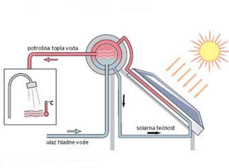
Sl.1.5. Pojednostavljeni prikaz korištenja solarnog panela za zagrijavanje vode [5]
